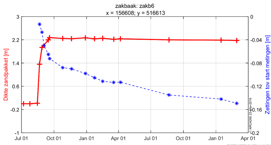
Figuur 6-38 Opgetreden zettingen in relatie met de dikte van het zandpakket in zakb6.
