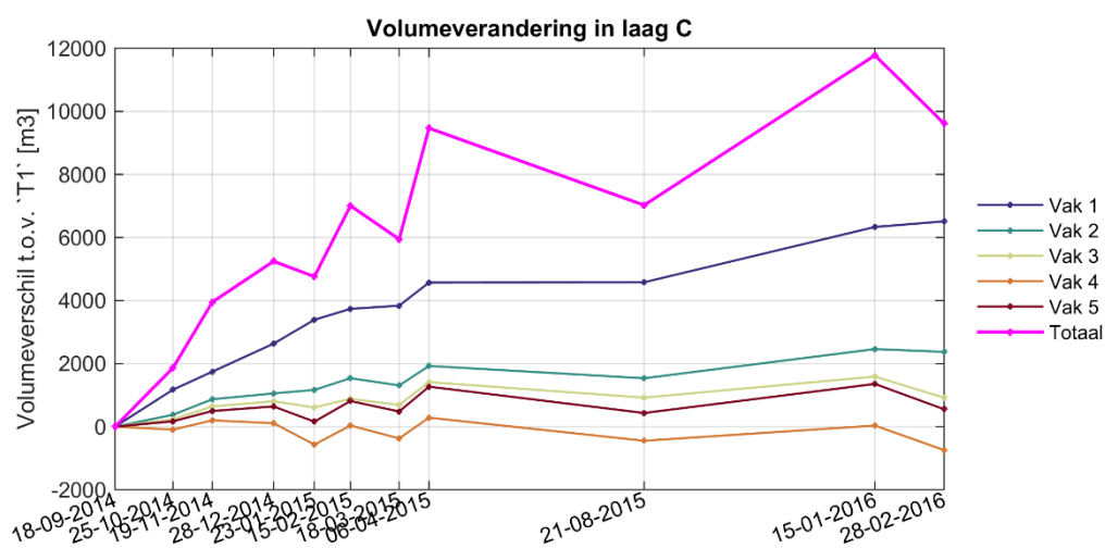
Figuur III - 2-18 Ontwikkeling volume onderlaag (C) per vak en gesommeerd over alle vakken.
