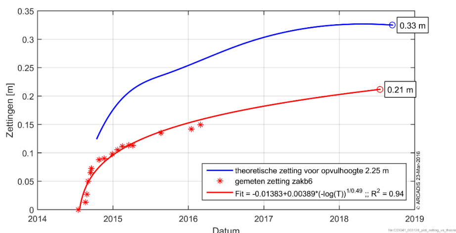
Figuur 6-48 Gemeten zettingen in zakb6 vergeleken met de theoretische zetting voor dit punt.
