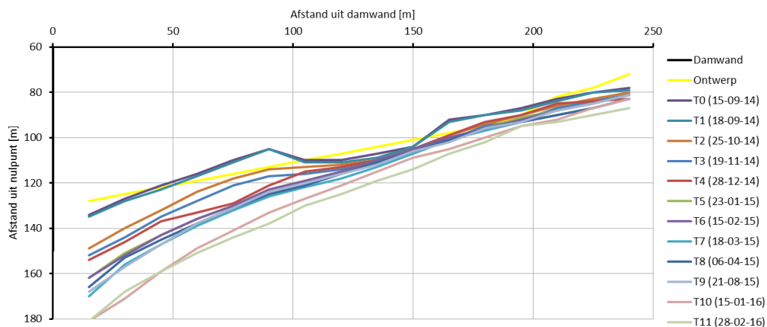
Figuur III - 2-10 Ontwikkeling positie onderlaag (positie doorsnijing op NAP-1,3 m) in centrale deel voor alle inmetingen.
