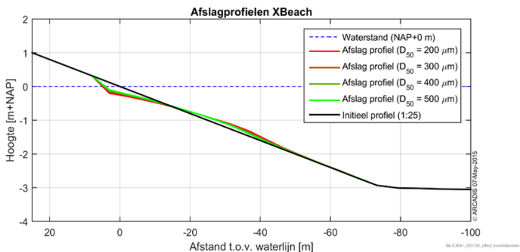
Figuur I - 3-2 Afhangelijkheid profielontwikkeling van korreldiameter voor XBEACH.
