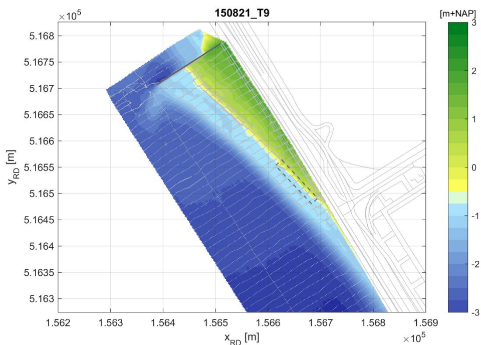
Figuur 6-10 Overzicht bodemligging T9 op 21 augustus 2015.
