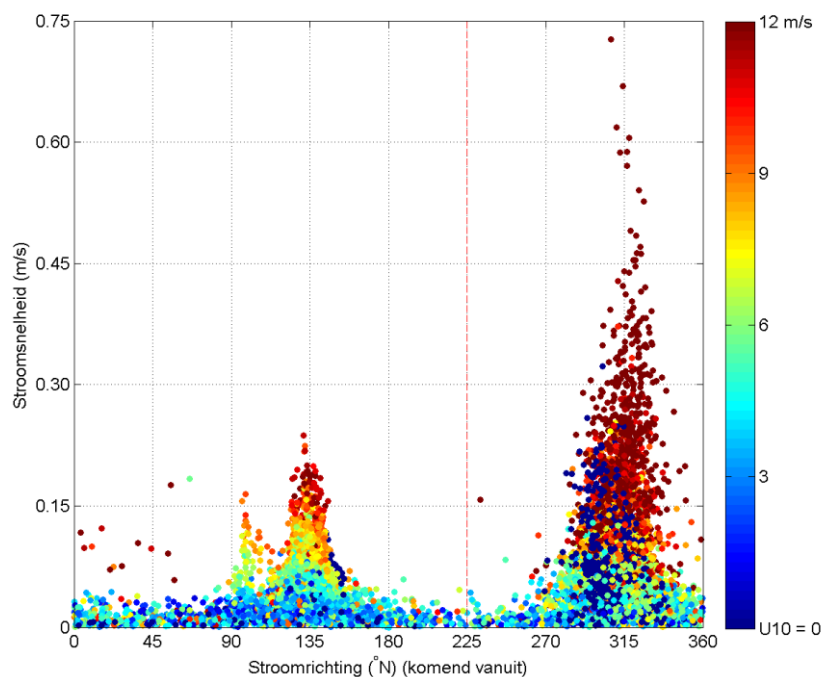
Figuur 5-18 Vergelijking stroomrichting (in graden ten opzichte van noord, gedefinieerd als 'komend vanuit') en stroomsnelheid (verticale as), waarbij de markers zijn gekleurd op windsnelheid.
