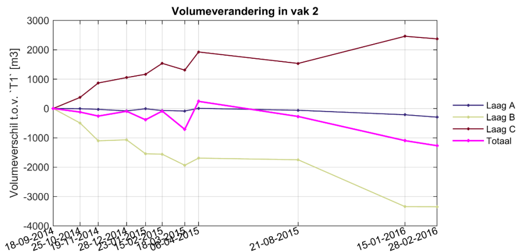
Figuur III - 2-21 Ontwikkeling volume vak2 per laag en gesommeerd over alle lagen.
