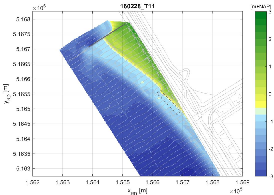
Figuur 6-12 Overzicht bodemligging T11 op 28 februari 2016.
