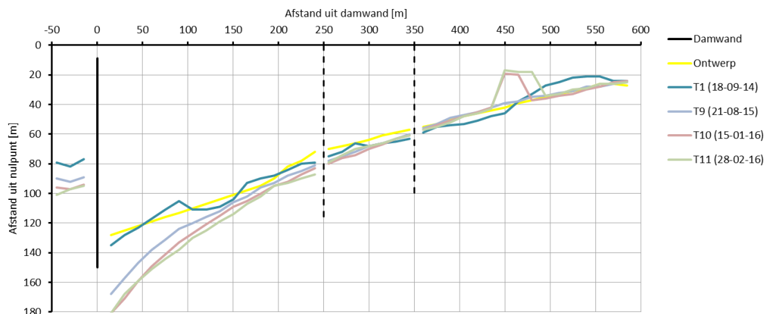
Figuur III - 2-9 Overzicht ontwikkeling positie onderlaag (positie doorsnijding op NAP-1,5 m) inclusief naastgelegen secties voor initiële en meest recente opnamen.
