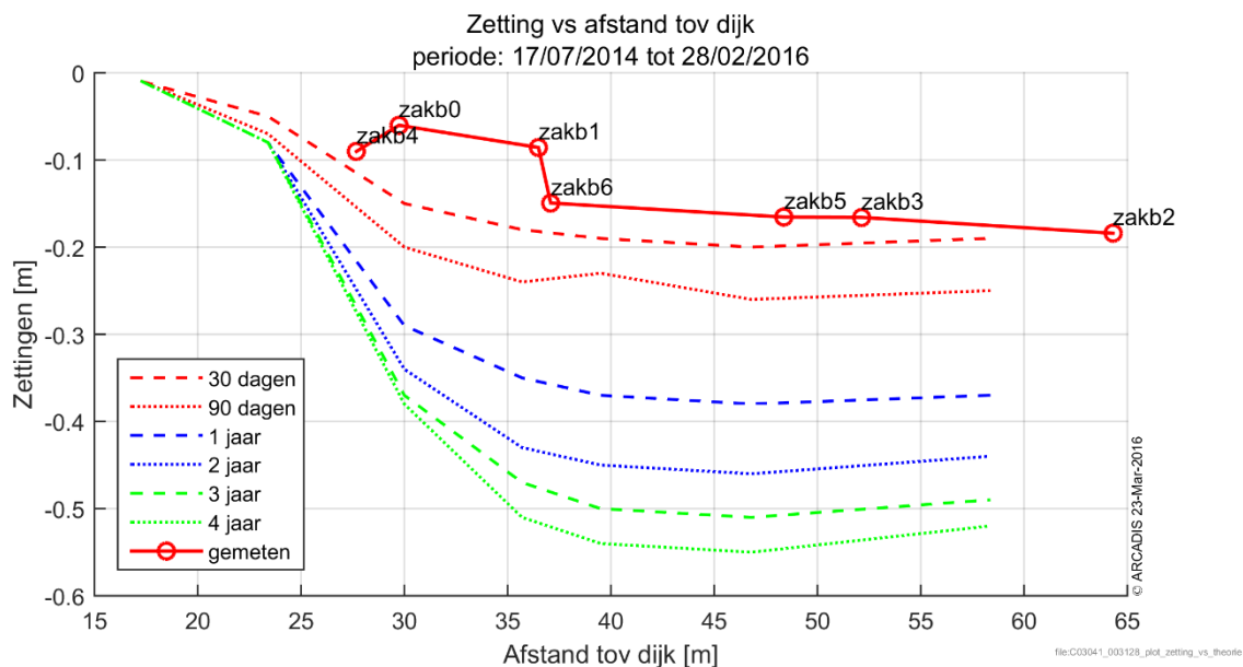
Figuur 6-41 Gemeten zettingen in kustdwarsrichting vergeleken met de voorspelde zettingen op meerdere momenten in de tijd.
