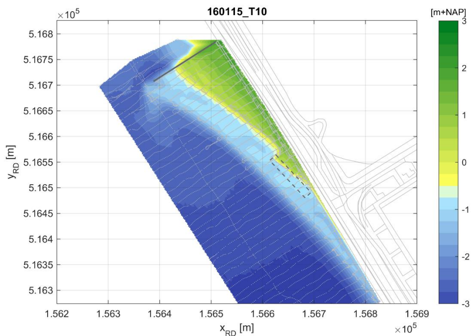
Figuur 6-11 Overzicht bodemligging T10 op 15 januari 2016.
