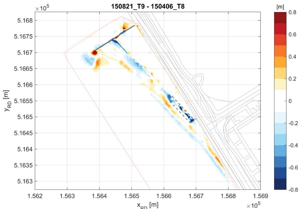
Figuur 6-21 Verschil in bodemligging tussen T8- en T9-opname.
