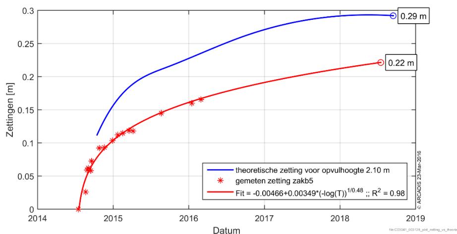
Figuur 6-47 Gemeten zettingen in zakb5 vergeleken met de theoretische zetting voor dit punt.
