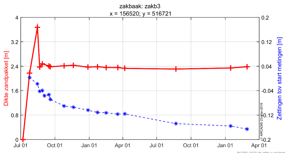
Figuur 6-35 Opgetreden zettingen in relatie met de dikte van het zandpakket in zakb3.
