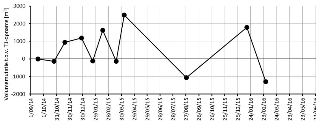
Figuur III - 2-11 Tijdsontwikkeling totaalvolume sinds start inmetingen (T1 op 18 september 2014).
