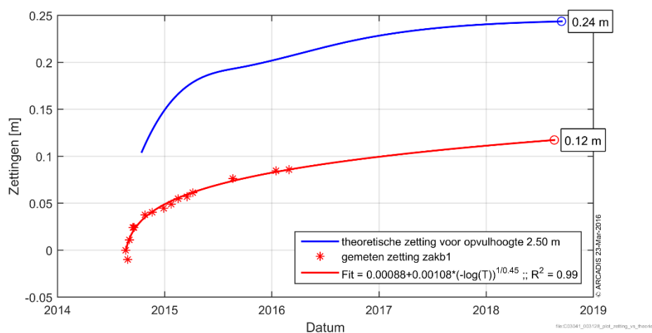
Figuur 6-43 Gemeten zettingen in zakb1 vergeleken met de theoretische zetting voor dit punt.
