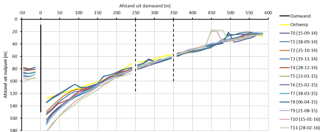
Figuur III - 2-8 Overzicht ontwikkeling positie onderlaag (positie doorsnijding op NAP-1,5 m) inclusief naastgelegen secties voor alle inmetingen.
