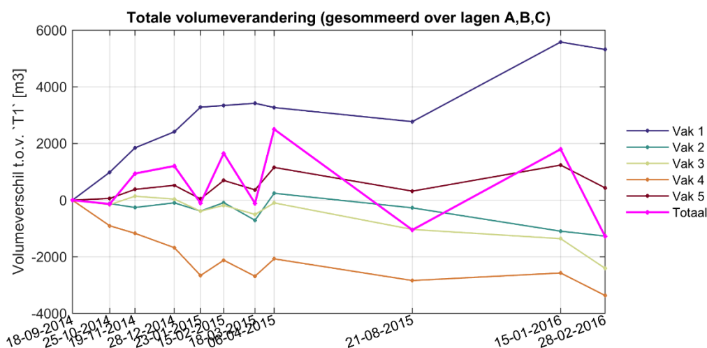
Figuur III - 2-19 Ontwikkeling volume per laag (A, B en C) en gesommeerd over alle lagen.
