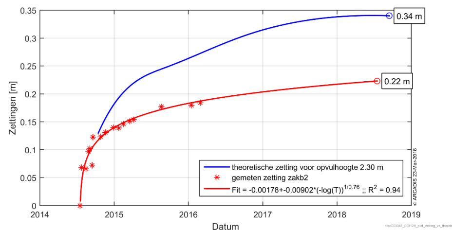
Figuur 6-44 Gemeten zettingen in zakb2 vergeleken met de theoretische zetting voor dit punt.
