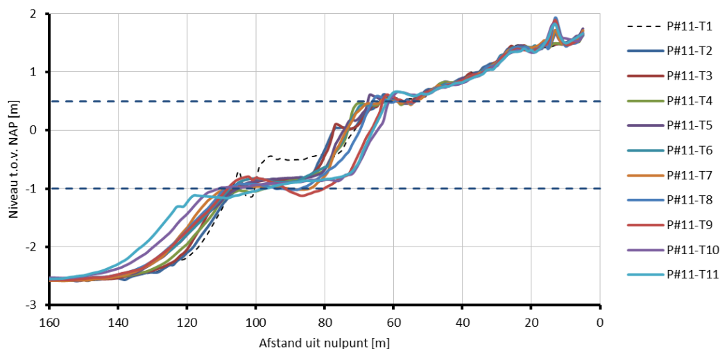
Figuur III - 2-13 Schematische weergave van de gehanteerde definities voor de bepaling van de verticale verdeling van de volume-vakken. Er is onderscheid gemaakt tussen 3 lagen: [A] boven NAP +0,5 m, [B] tussen NAP -1 m en NAP +0,5 m, [C] onder NAP -1 m.
