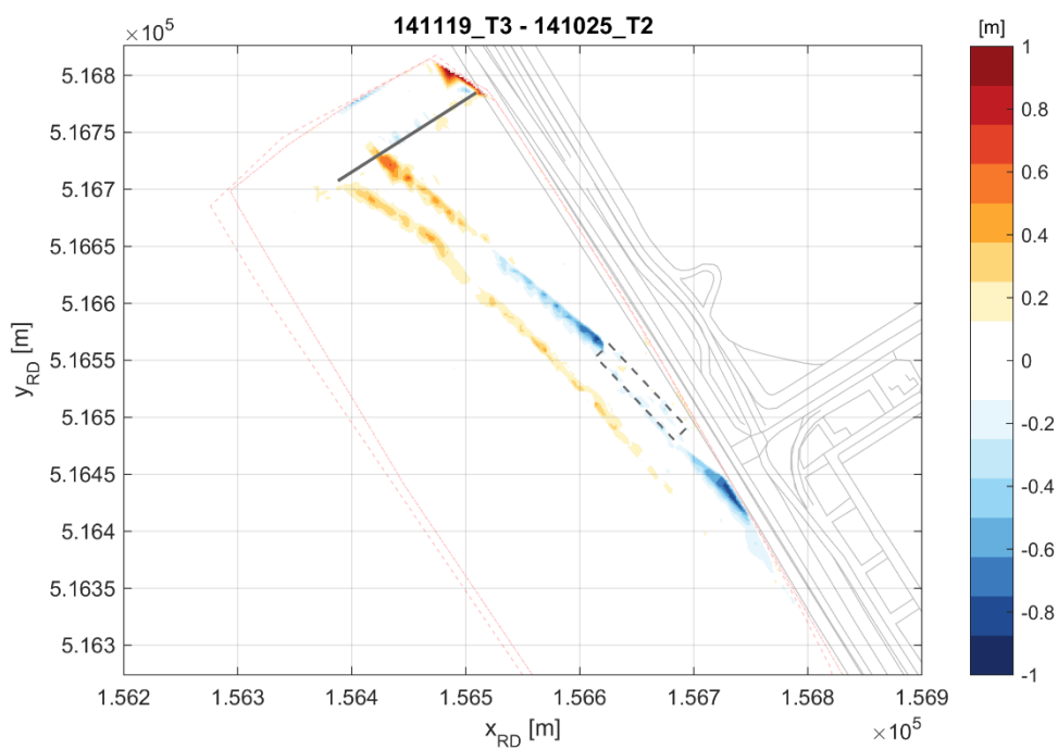
Figuur 6-15 Verschil in bodemligging tussen T2- en T3-opname.
