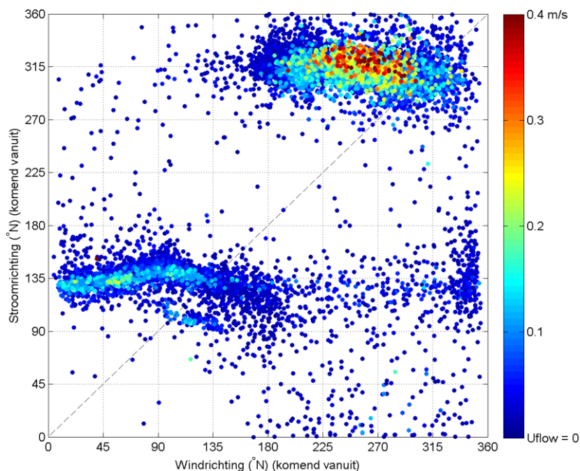
Figuur 5-19 Vergelijking windrichting (horizontale as) en stroomrichting (verticale as, beide in graden ten opzichte van noord, gedefinieerd als 'komend vanuit'), waarbij de markers zijn gekleurd op stroomsnelheid in m/s. Stroomsnelheden onder 0.01 m/s zijn niet weergegeven.
