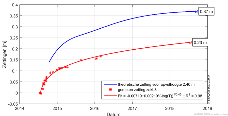
Figuur 6-45 Gemeten zettingen in zakb3 vergeleken met de theoretische zetting voor dit punt.
