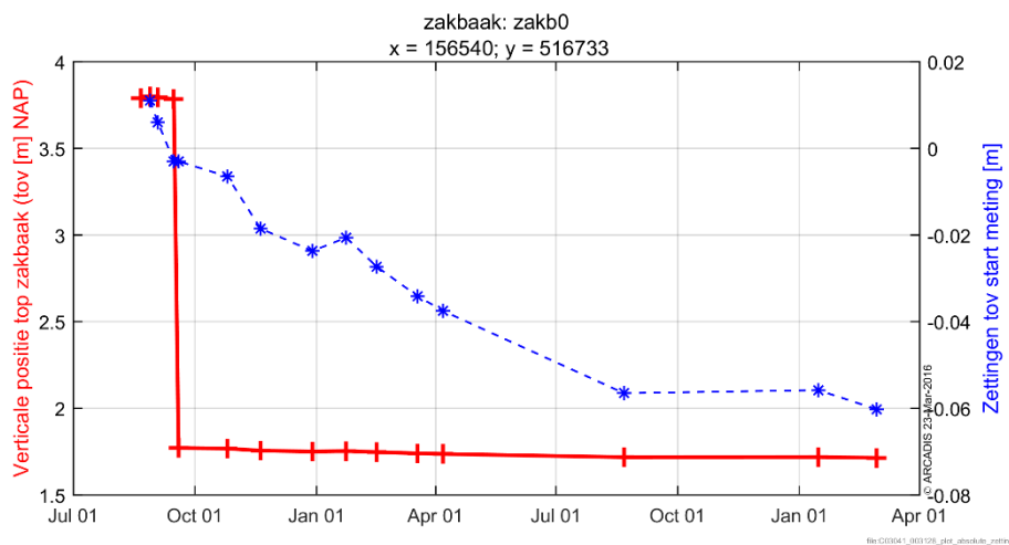
Figuur 6-25 Absolute ontwikkeling top van het zakkaken voor zakb0 (rode lijn), samen met de bijbehorende zetting (blauwe lijn).
