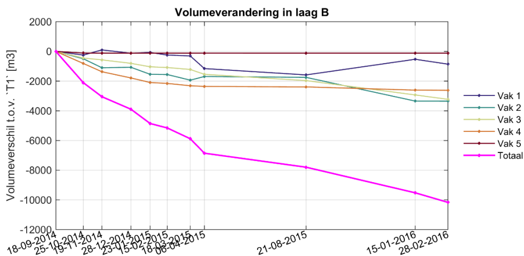
Figuur III - 2-17 Ontwikkeling volume oeverlaag (B) per vak en gesommeerd over alle vakken.
