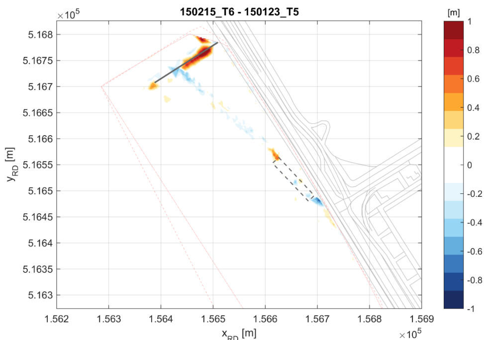
Figuur 6-18 Verschil in bodemligging tussen T5- en T6-opname.
