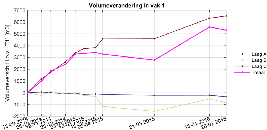
Figuur III - 2-20 Ontwikkeling volume vak1 per laag en gesommeerd over alle lagen.
