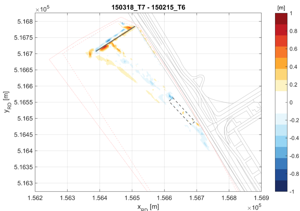
Figuur 6-19 Verschil in bodemligging tussen T6- en T7-opname.
