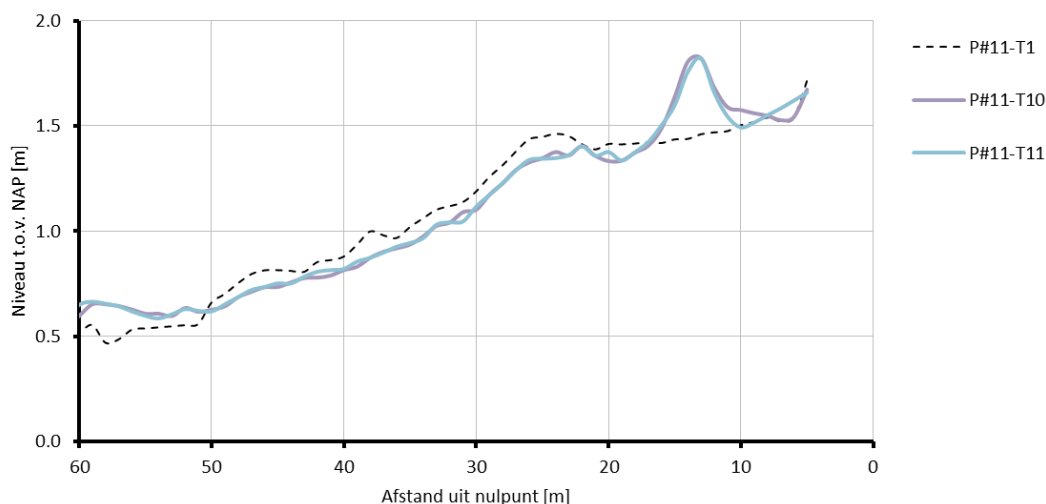
Figuur III - 2-12 Vergelijking initiële en meest recente bodemligging ter plaatse van profiel #11 op 120 m uit de damwand voor het droge deel van de proefsectie.
