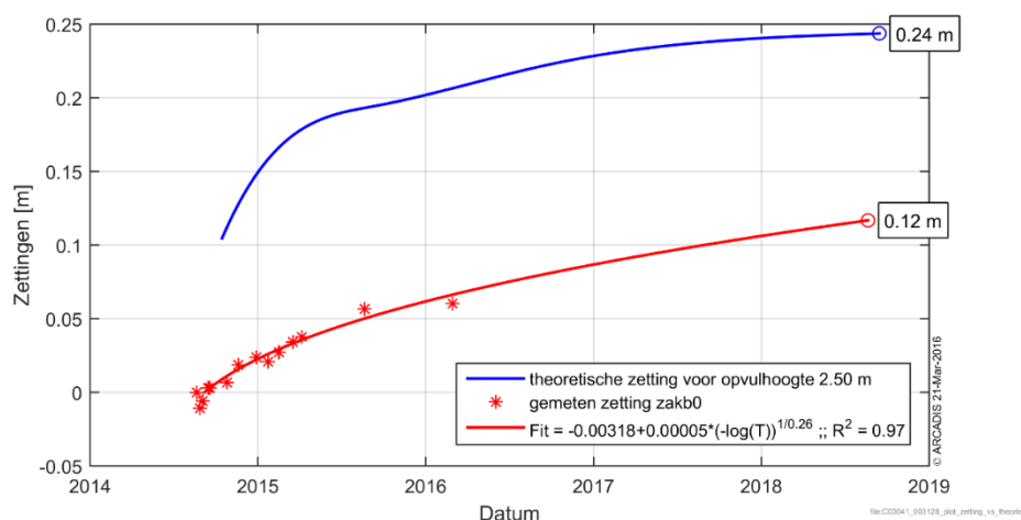
Figuur 6-42 Gemeten zettingen in zakb0 vergeleken met de theoretische zetting voor dit punt.
