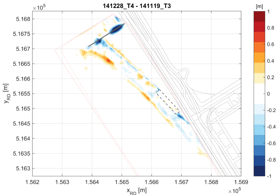
Figuur 6-16 Verschil in bodemligging tussen T3- en T4-opname.
