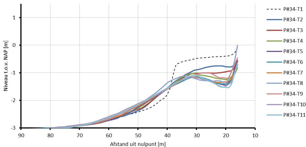
Figuur III - 2-25 Overzicht profielontwikkeling in profiel #34 op 465 m uit de damwand.
