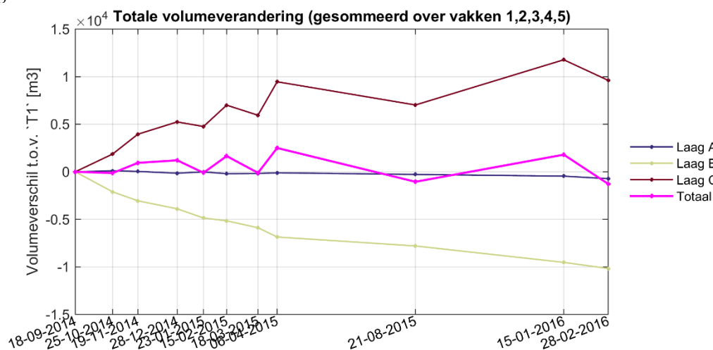
Figuur III - 2-15 Ontwikkeling volume per laag (A, B en C) en gesommeerd over alle lagen.
