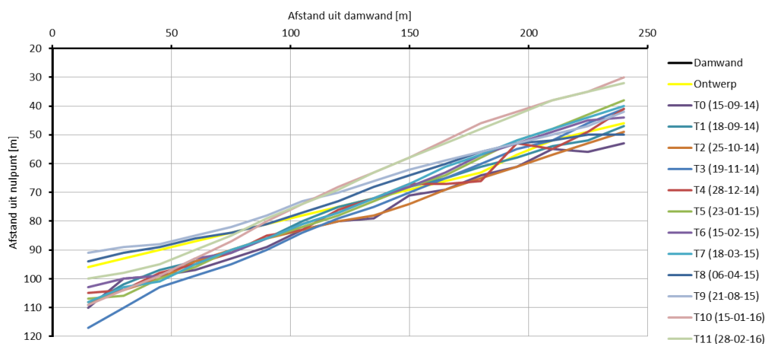
Figuur III - 2-4 Detail positie oeverlijn over centrale deel proefsectie (tussen damwand en rijsmatconstructie).
