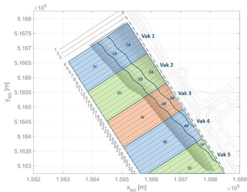
Figuur III - 2-14 Schematisch overzicht van de gehanteerde indeling van volume-vakken in het studiegebied. De rechte lijnen geven aan dat de begrenzingen van het betreffende vak 'geografisch' zijn bepaald, en de golvende lijnen geven aan dat de begrenzingen zijn bepaald op basis van verticale niveaus (en dus afhankelijk zijn van de profiellegging).
