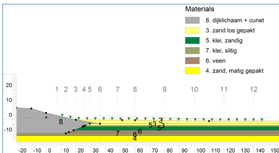
Figuur 6-39 Schematisatie ondergrond Houtribdijk ter plaatse van pilot.
