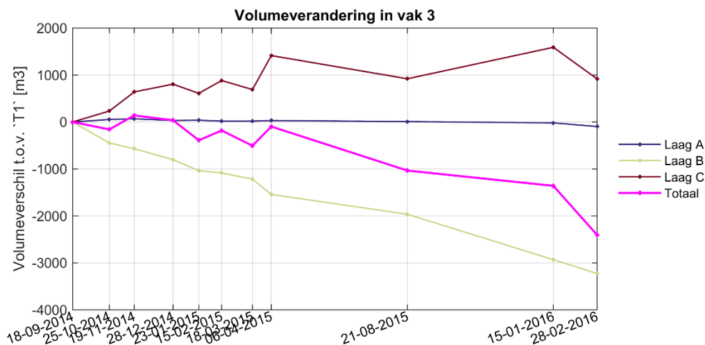
Figuur III - 2-22 Ontwikkeling volume vak 3 (rijmatconstructie) per laag en gesommeerd over alle lagen.
