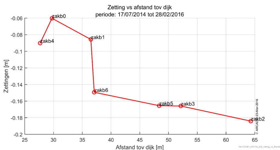
Figuur 6-40 Gemeten zettingen uitgezet tegen de afstand in kustdwarsrichting.
