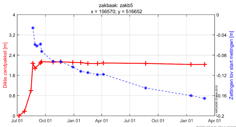
Figuur 6-37 Opgetreden zettingen in relatie met de dikte van het zandpakket in zakb5.
