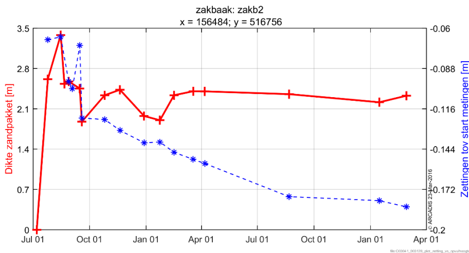
Figuur 6-34 Opgetreden zettingen in relatie met de dikte van het zandpakket in zakb2.
