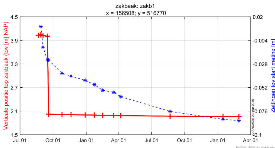
Figuur 6-26 Absolute ontwikkeling top van het zakkaken voor zakb1 (rode lijn), samen met de bijbehorende zetting (blauwe lijn).
