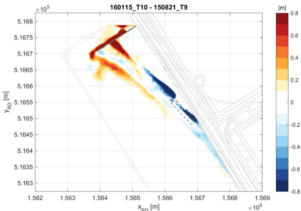
Figuur 6-22 Verschil in bodemligging tussen T9- en T10-opname.
