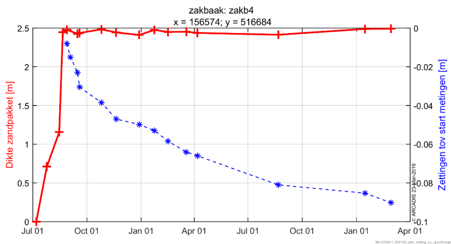
Figuur 6-36 Opgetreden zettingen in relatie met de dikte van het zandpakket in zakb4.
