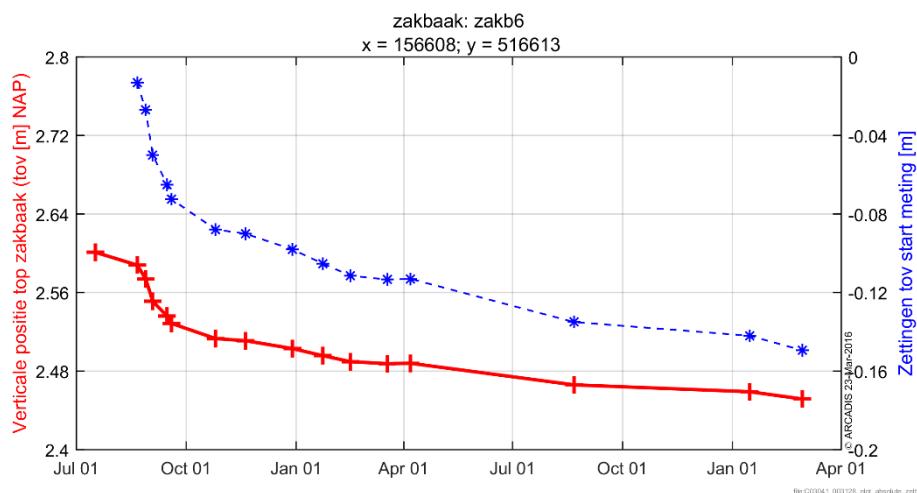
Figuur 6-31 Absolute ontwikkeling top van het zakbaken voor zakb6 (rode lijn), samen met de bijbehorende zetting (blauwe lijn).
