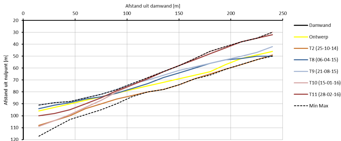
Figuur III - 2-5 Overzicht variatie in oeverlijnposities in centrale deel proefsectie.
