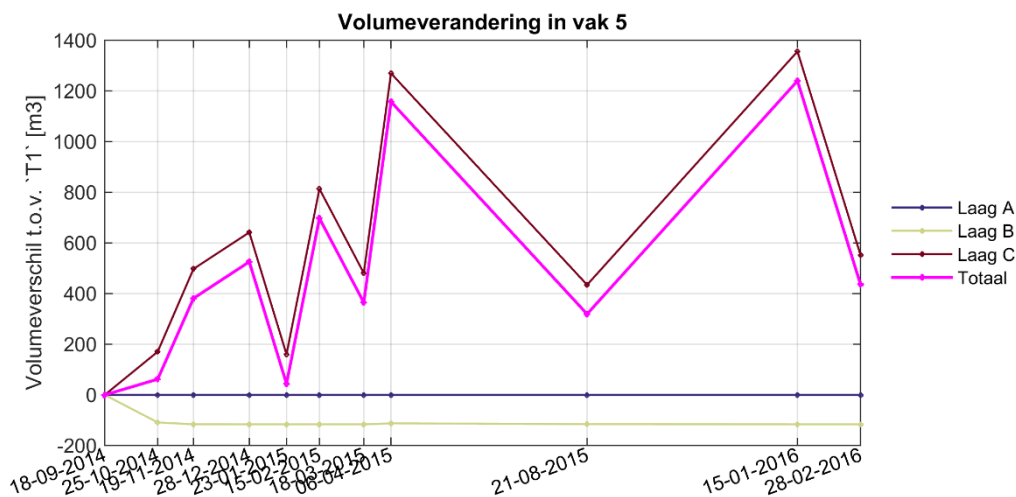
Figuur III - 2-24 Ontwikkeling volume vak 5 per laag en gesommeerd over alle lagen.
