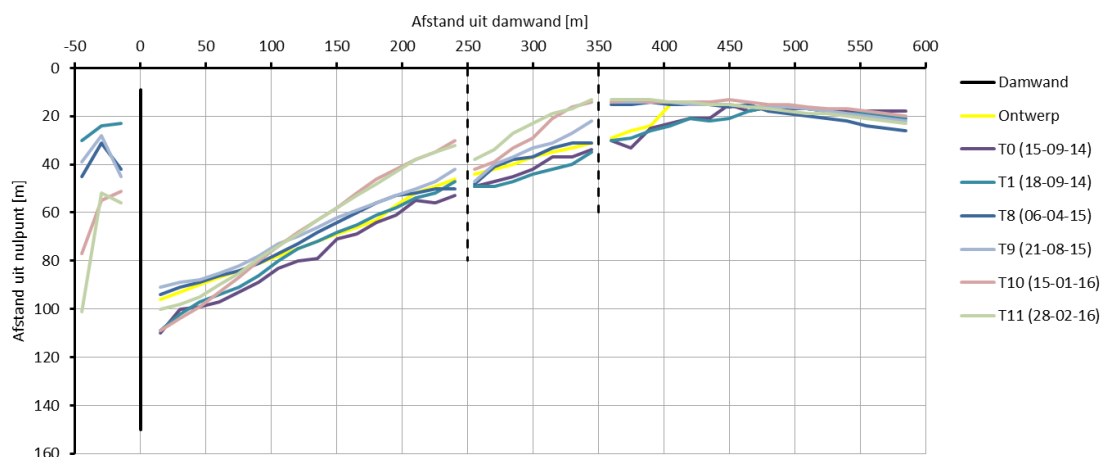
Figuur III - 2-3 Overzicht ontwikkeling positie oeverlijn (positie doorsnijding op NAP-0,3 m) inclusief naastgelegen secties voor relevante inmetingen.
