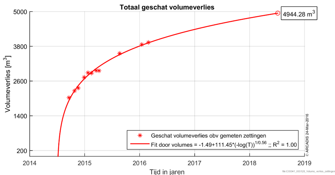
Figuur 6-49 Geschat verloop van het zetting gerelateerd volumeverlies.
