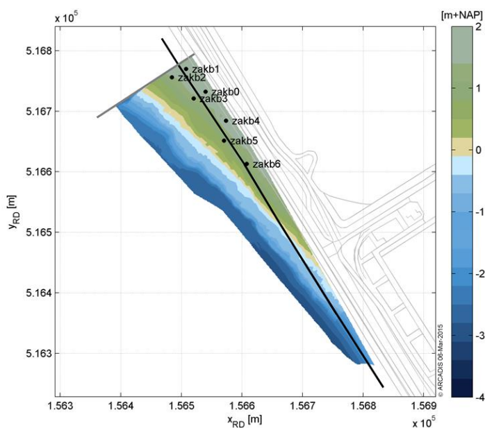
Figuur 6-24 Overzicht positie van de zeven geplaatste zakbakens, inclusief de begrenzing van het cunet (zwarte lijn).
