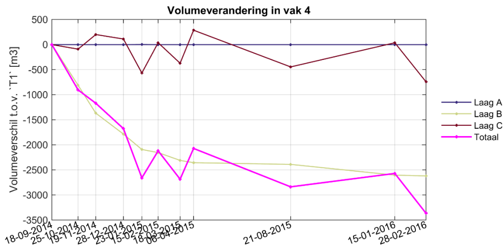
Figuur III - 2-23 Ontwikkeling volume vak 4 per laag en gesommeerd over alle lagen.
