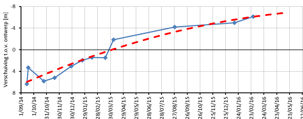
Figuur III - 2-7 Tijdsontwikkeling ligging positie zwaartepunt centrale proefsectie.
