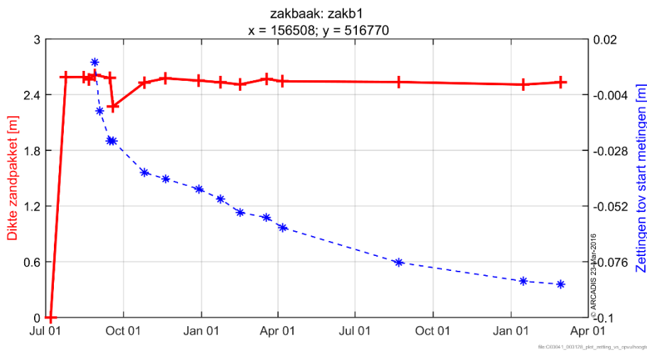
Figuur 6-33 Opgetreden zettingen in relatie met de dikte van het zandpakket in zakb1.
