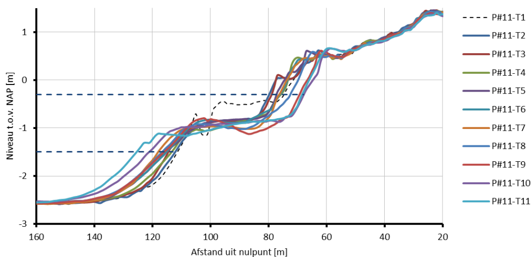
Figuur III - 2-1 Ontwikkeling dwarsprofiel in profiel #11 (op 120 m uit damwand) met daarin aangegeven de gehanteerde niveaus voor het bepalen van de karakteristieke posities van oeverlijn (NAP-0,3 m) en onderlaag (NAP-1,5 m).
