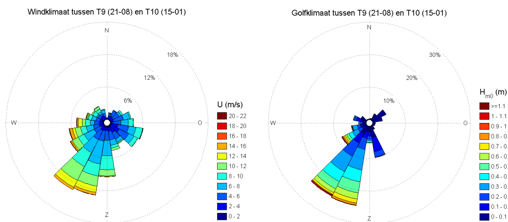
Figuur 5-30 Wind- en golfklimaat tussen T9 en T10.
