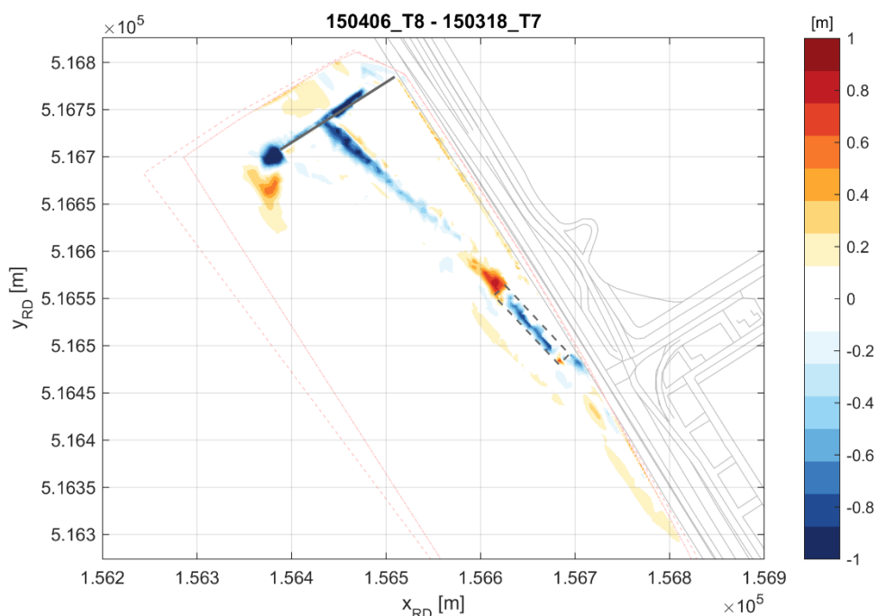
Figuur 6-20 Verschil in bodemligging tussen T7- en T8-opname.
