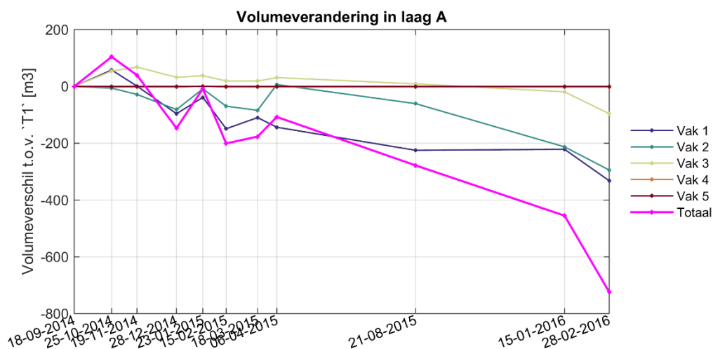
Figuur III - 2-16 Ontwikkeling volume bovenlaag (A) per vak en gesommeerd over alle vakken.
