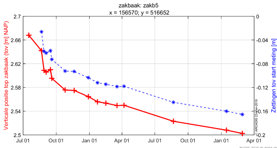
Figuur 6-30 Absolute ontwikkeling top van het zakbaken voor zakb5 (rode lijn), samen met de bijbehorende zetting (blauwe lijn).
