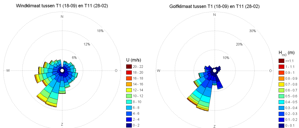
Figuur 5-21 Wind- en golfklimaat hele meetinterval tussen T1 en T11.
