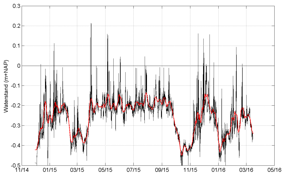
Figuur 5-4 Gemeten waterstand (zwart) en een lopend gemiddelde met een middellingsperiode van een week (rood).
