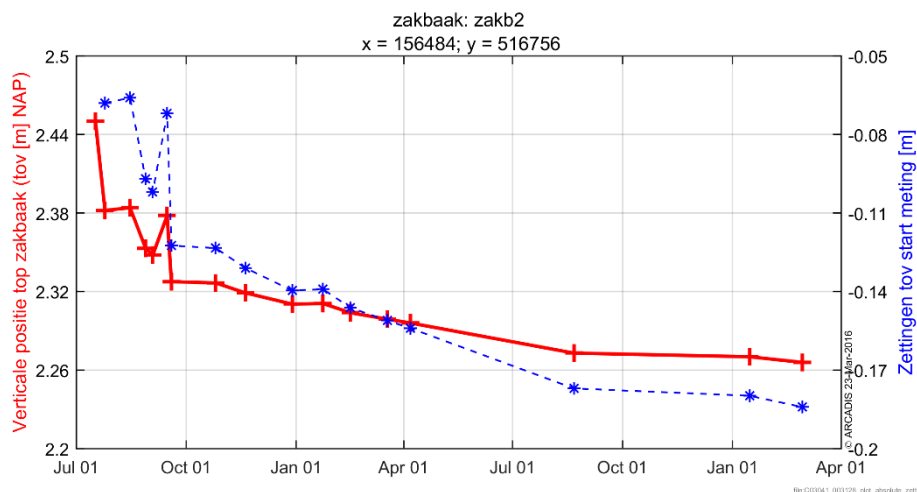
Figuur 6-27 Absolute ontwikkeling top van het zakbaken voor zakb2 (rode lijn), samen met de bijbehorende zetting (blauwe lijn).
