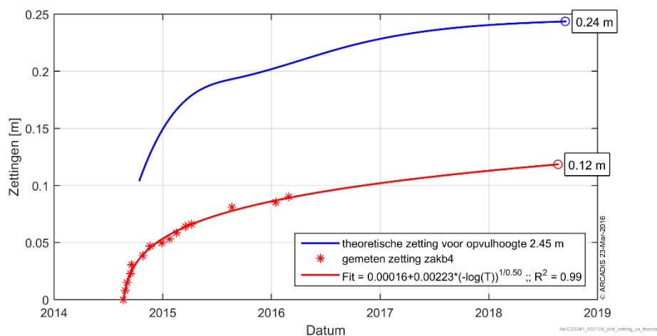
Figuur 6-46 Gemeten zettingen in zakb4 vergeleken met de theoretische zetting voor dit punt.
