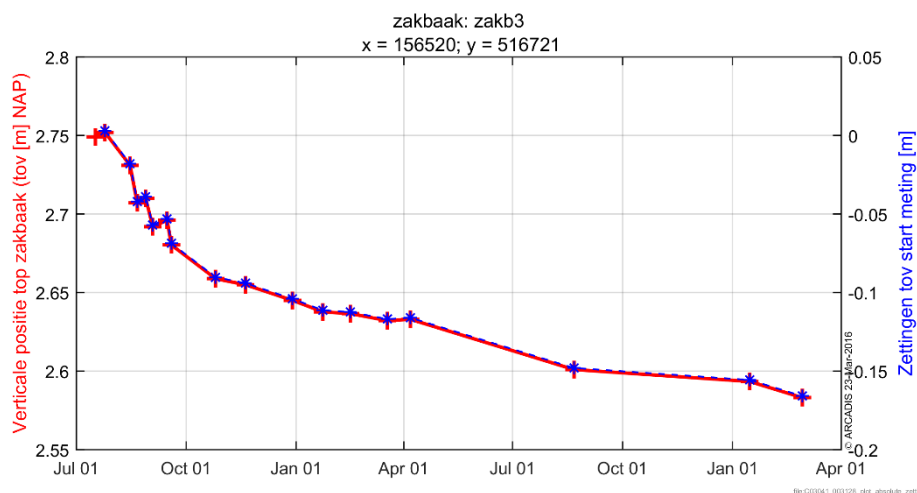
Figuur 6-28 Absolute ontwikkeling top van het zakbaken voor zakb3 (rode lijn), samen met de bijbehorende zetting (blauwe lijn).
