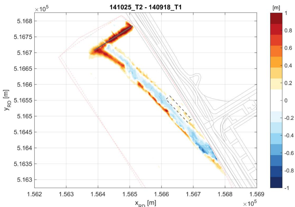
Figuur 6-14 Verschil in bodemligging tussen T1- en T2-opname.
