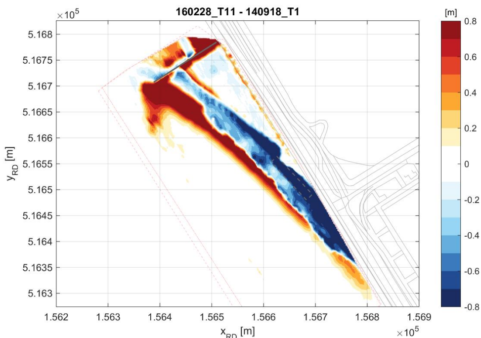
Figuur 6-13 Verschillen in bodemligging tussen eerste en laatste inmeting (T11).
