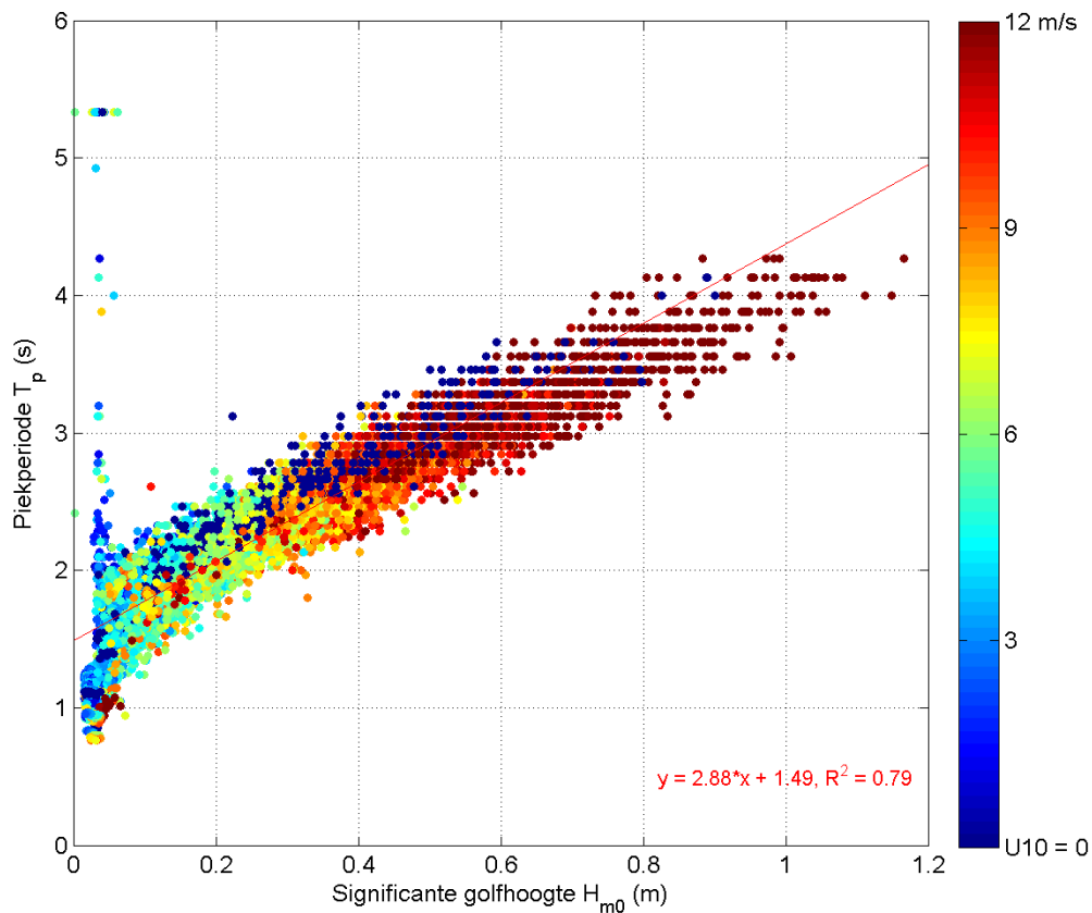
Figuur 5-15 Vergelijking significante golfhoopte H_{m0} (horizontale as) en piekperiode T_p (verticale as), waarbij de markers zijn gekleurd op windsnelheid.
