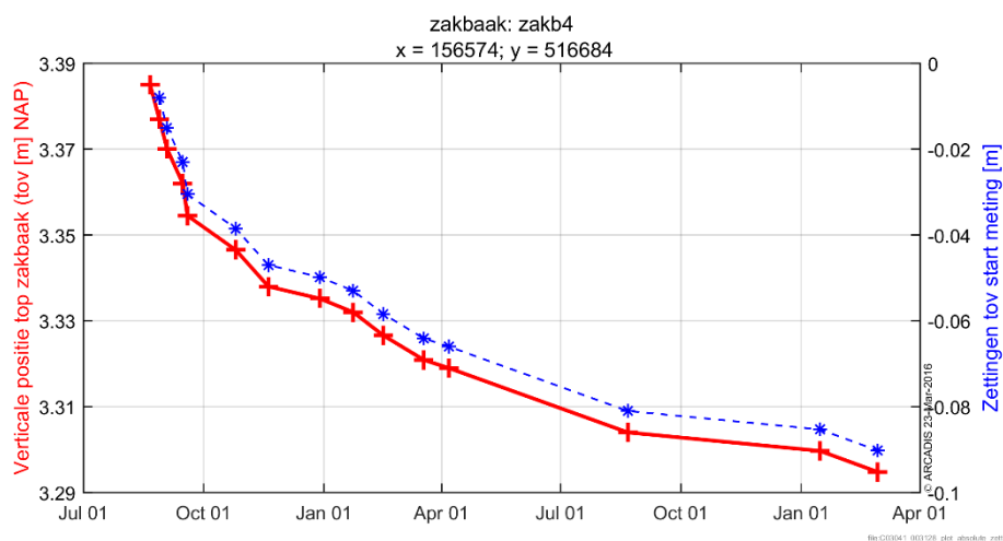
Figuur 6-29 Absolute ontwikkeling top van het zakbaken voor zakb4 (rode lijn), samen met de bijbehorende zetting (blauwe lijn).
