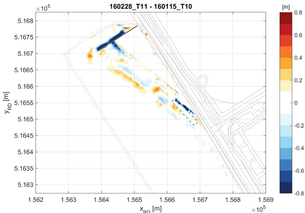
Figuur 6-23 Verschil in bodemligging tussen T10- en T11-opname.
