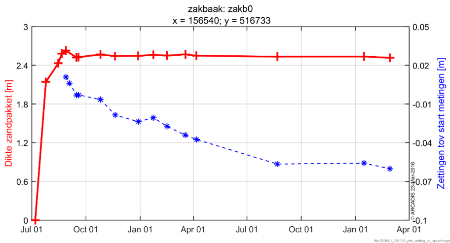
Figuur 6-32 Opgetreden zettingen in relatie met de dikte van het zandpakket in zakb0.
