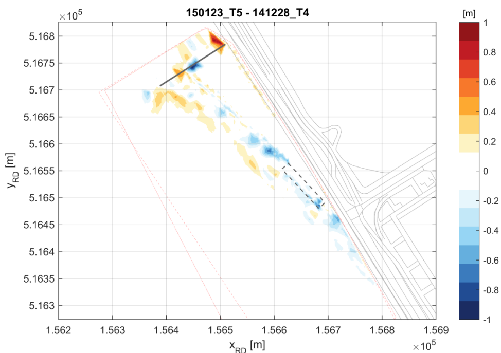
Figuur 6-17 Verschil in bodemligging tussen T4- en T5-opname.
