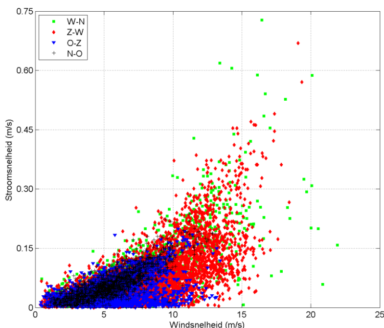
Figuur 5-20 Vergelijking windsnelheid (horizontale as) en stroomsnelheid (verticale as) voor vier verschillende windsectoren
